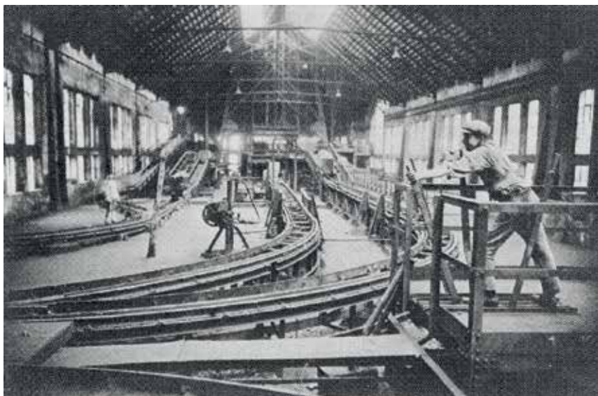
Een beeld van de losvloer. Kettingbanen zorgen voor een automatische omloop van volle en lege wagens.
